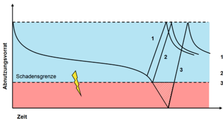
Abb. 2 Abbau des Abnutzungsvorrats
